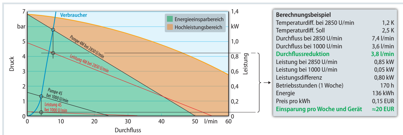
Bild 3. Die Beispielergebnisse zeigen: Das Zulassen einer doppelten Temperaturdifferenz bringt eine Durchflussreduktion von 7,4 l/min auf 3,6 l/min. Daraus ergibt sich eine wöchentliche Einsparung von 136 kWh, was bei einem Preis von 0,15 Euro pro kWh eine um 20 Euro geringere wöchentliche Stromrechnung bedeutet – bei nur einem Gerät. Quelle: HB-Therm; Grafik: © Hanser
