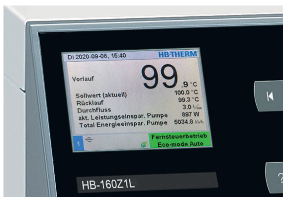
Bild 2. Im Klartext: Auf dem Bildschirm eines Thermo-5 mit Eco-pump erscheinen sowohl Sollwert als auch Rücklauftemperatur, die Durchflussmenge sowie die aktuelle Leistungseinsparung und die insgesamt eingesparte Energie pro Gerät (links). Die Werte zur Leistungsoptimierung wurden während eines Versuchs zur Serienfertigung einer Blende (rechts) in Wieselburg ermittelt © ZKW
